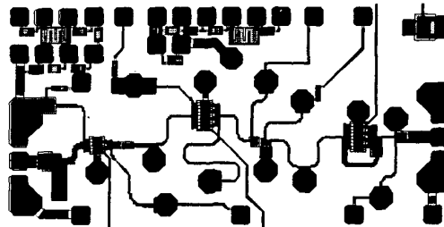
Fig. 8. LNA MMIC layout.
